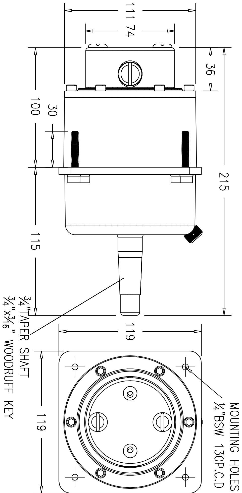
Dimensions - Model 101-102
